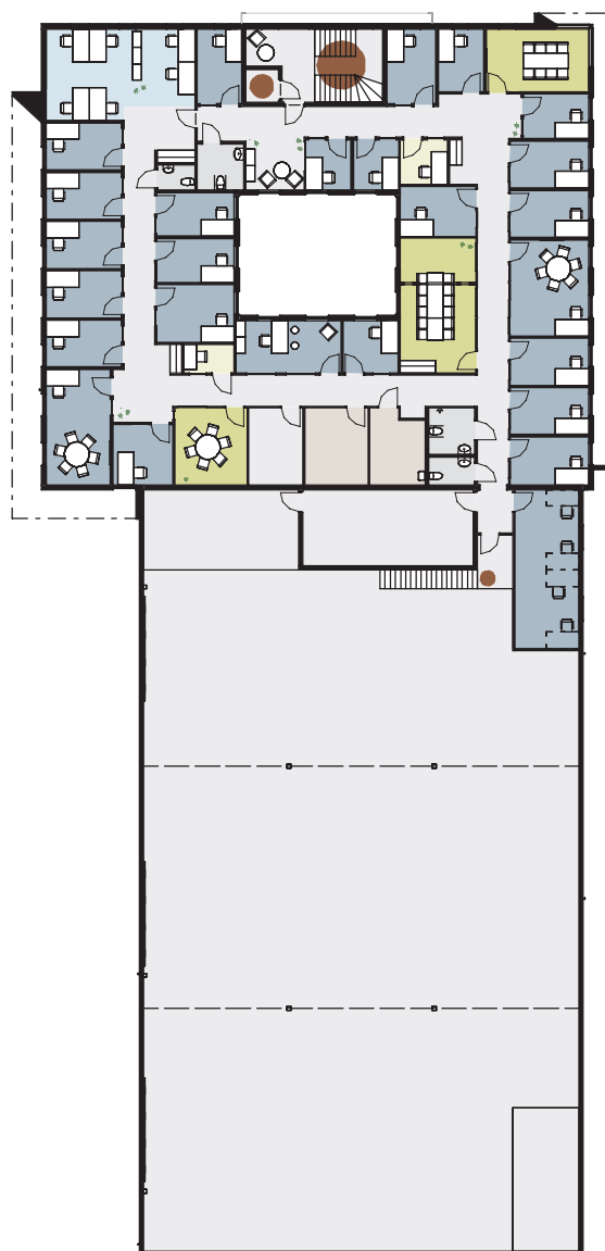
VÅNING 2
